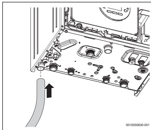
Fig. 22 Montar la manguera en el sifón de condensado
