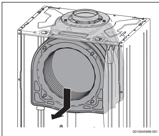
Fig. 102 Retirar el intercambiador de calor
