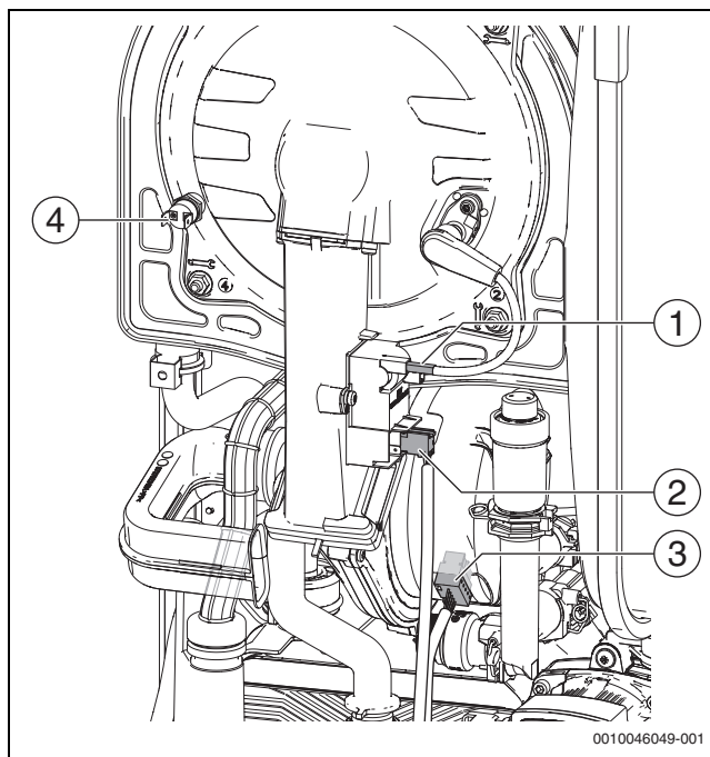
Fig. 126 Conectar el cable
