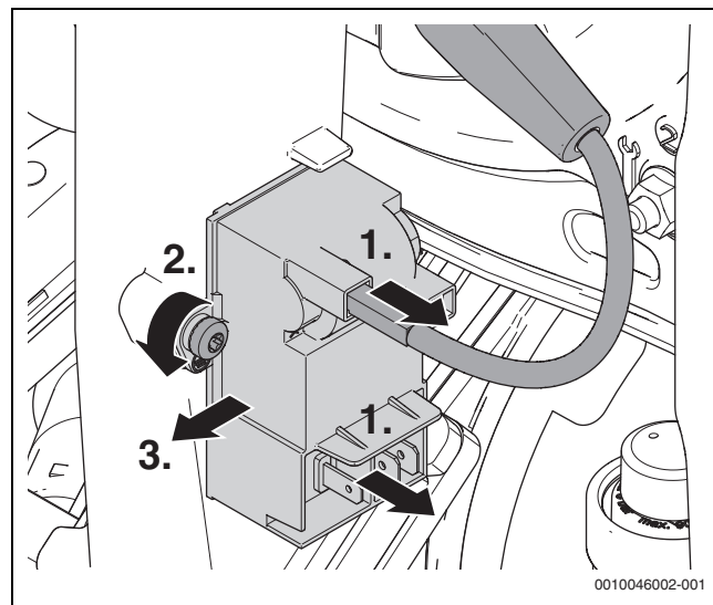
Fig. 105 Desmontar el transformador de encendido
