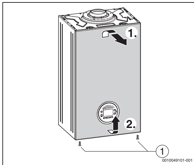
Fig. 39 Retirar la carcasa frontal
