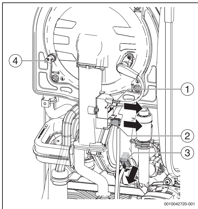
Fig. 40 Desconectar la conexión eléctrica
