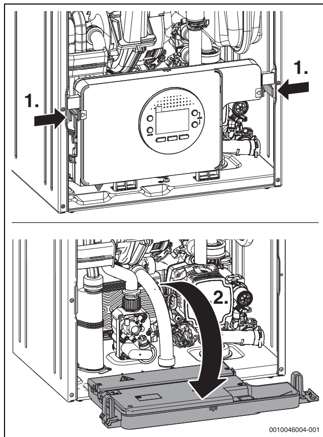
Fig. 27 Plegar la electrónica hacia abajo
