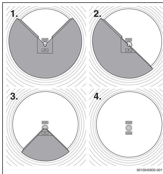
Fig. 70 Pasos para el desmontaje del aislamiento
