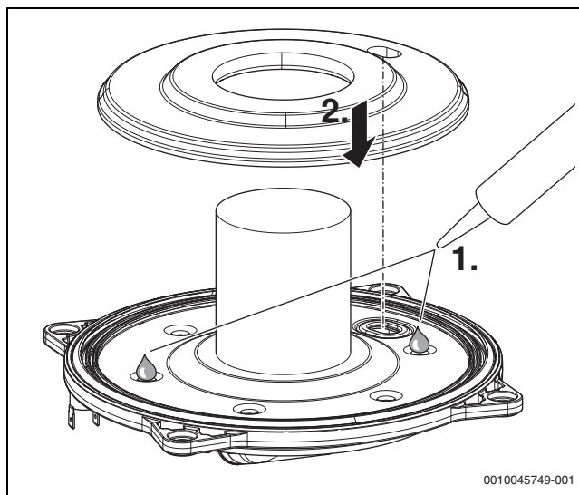
Fig. 65 Aplicar pegamento de silicona y colocar el nuevo aislamiento
