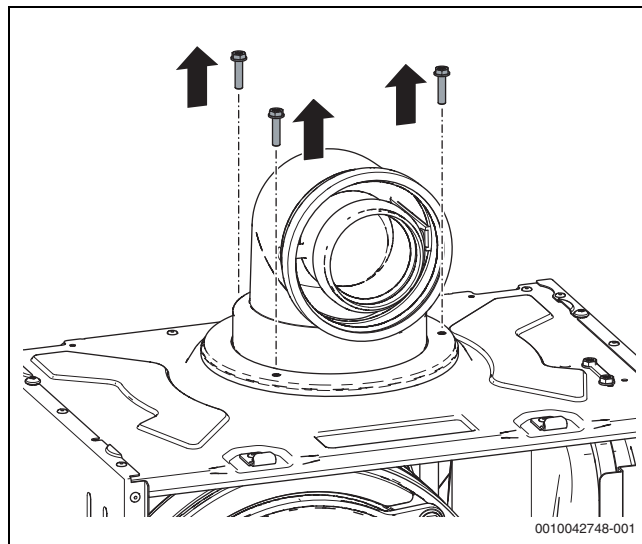
Fig. 145 Retirar los tornillo de sujeción
