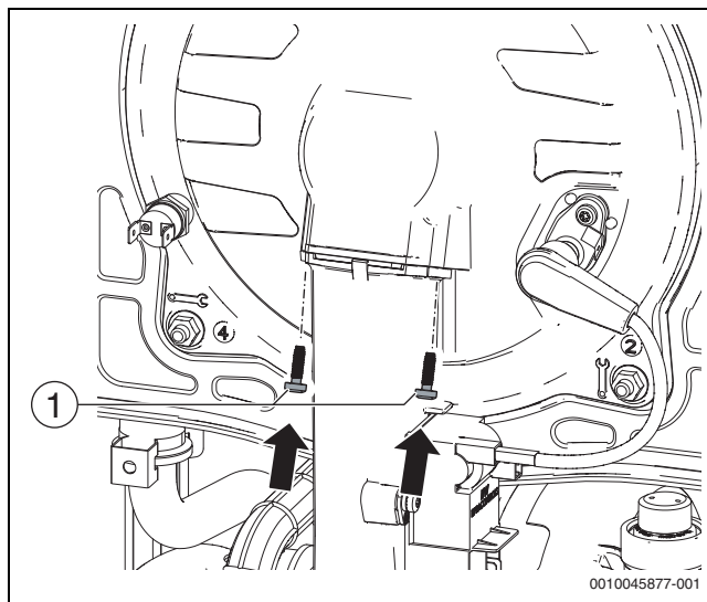
Fig. 79 Montaje de los tornillos en la puerta de la cámara de combustión
