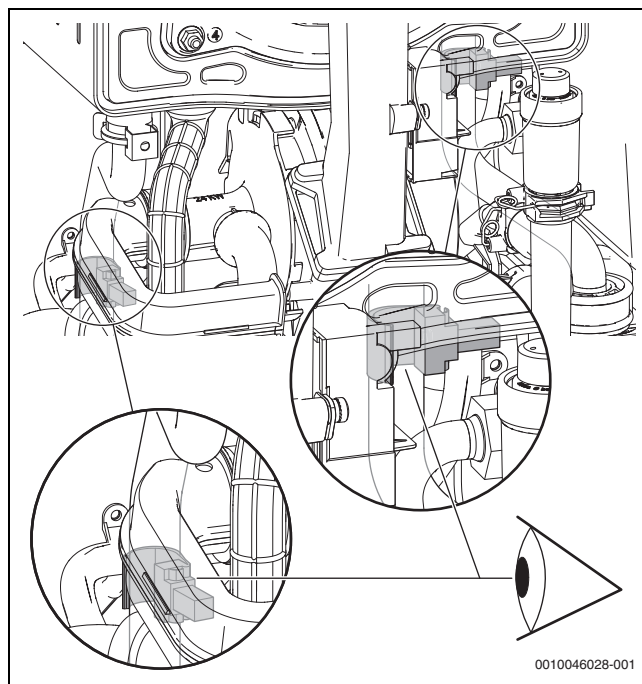
Fig. 54 Posición NTC
