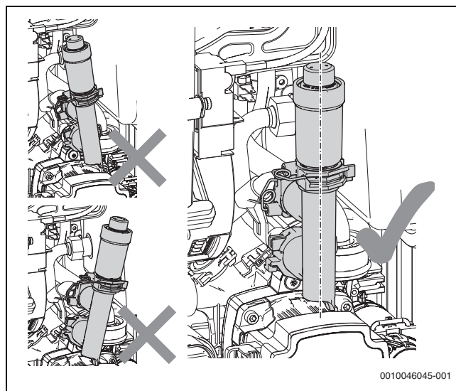
Fig. 130 Posición del purgador de aire
