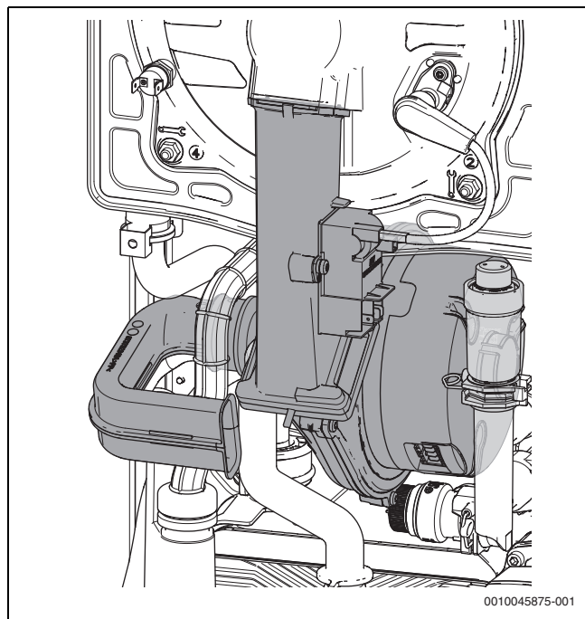
Fig. 77 Desmontaje de los componentes
