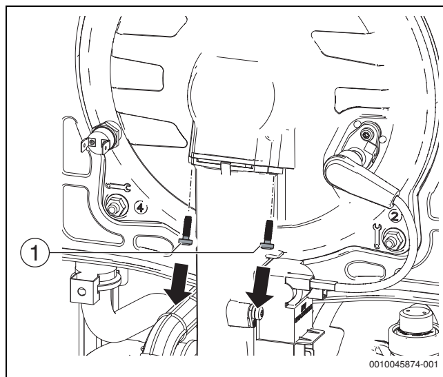
Fig. 114 Desmontaje de los tornillos
