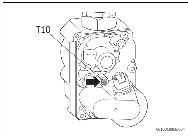
Fig. 37 Racor de medición para la presión de conexión de gas
