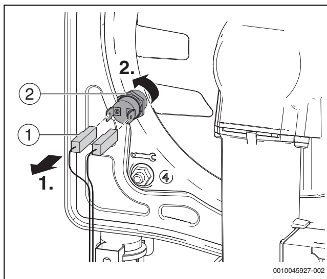
Fig. 94 Desmontaje del limitador de temperatura
