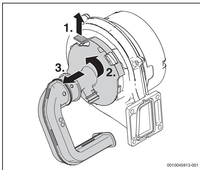
Fig. 87 Desmontaje del ventilador
