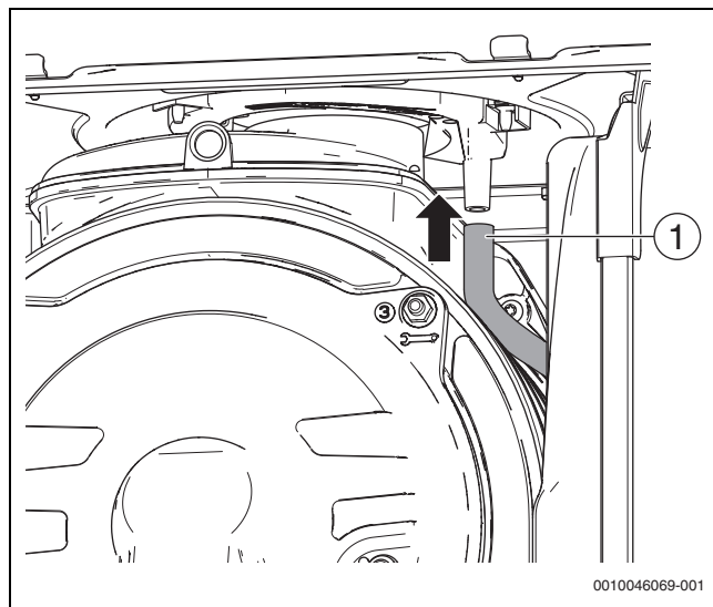
Fig. 61 Instalar la manguera de salida de agua
