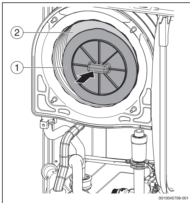
Fig. 45 Protección de aislamiento
