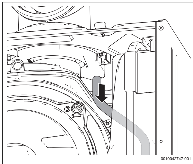
Fig. 144 Desmontar la protección contra la lluvia
