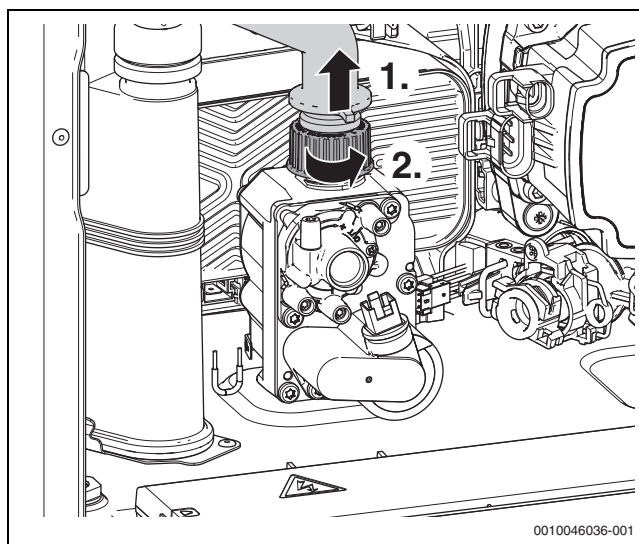
Fig. 118 Desmontar la manguera de conexión de gas y la tuerca de gas
