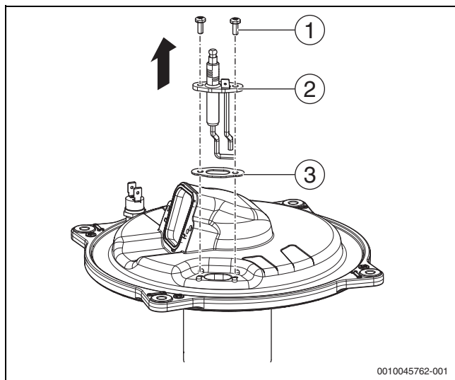
Fig. 66 Desmontaje del electrodo de encendido
