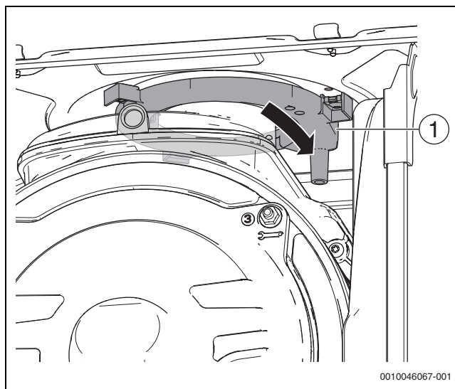
Fig. 58 Desmontar la protección contra las lluvias
