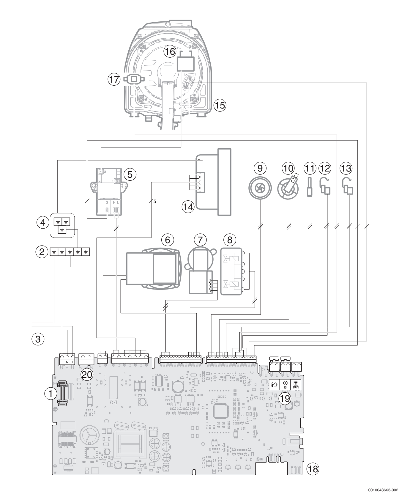
Fig. 153 Cableado eléctrico
