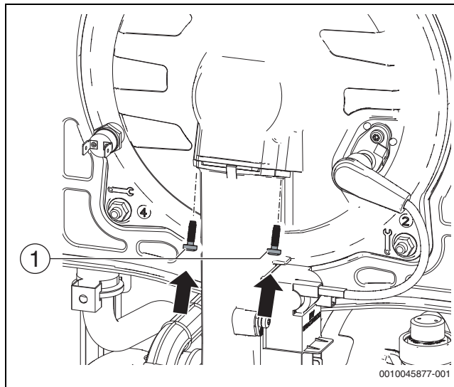
Fig. 117 Montaje de los tornillos en la puerta de la cámara de combustión
