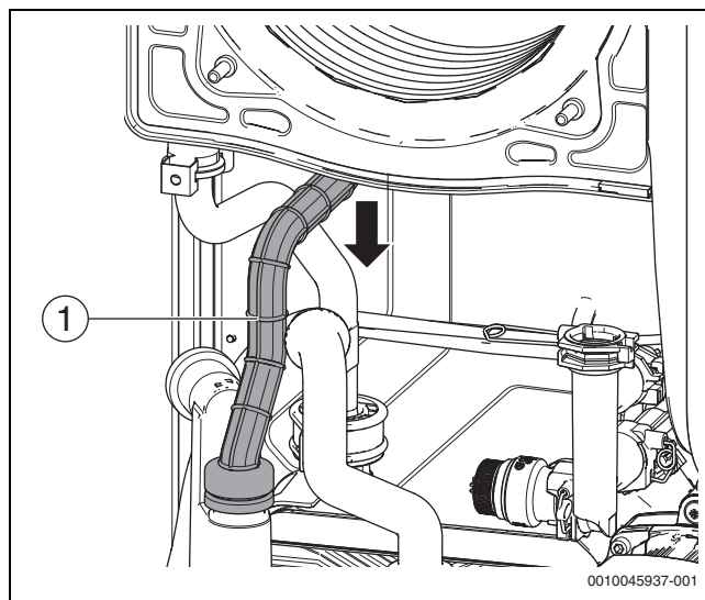
Fig. 98 Soltar el tubo de purga de condensados
