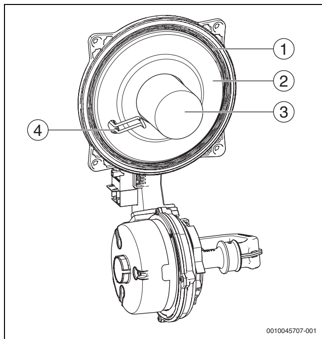
Fig. 44 Módulo de puerta de cámara de combustión
