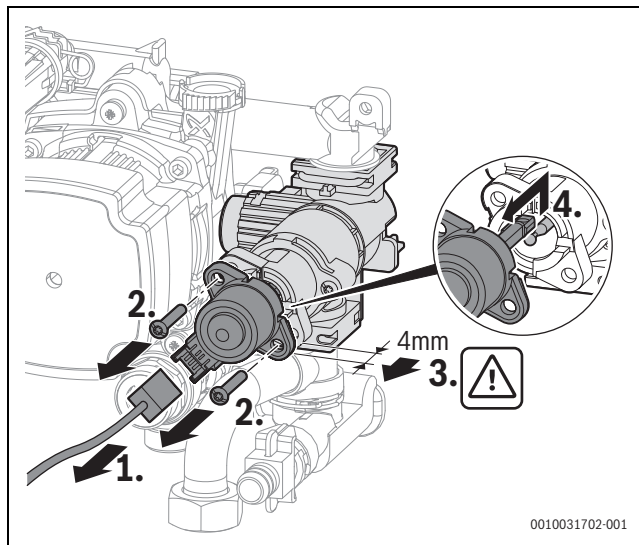
Fig. 149 Desmontar el motor en la válvula de 3 vías
