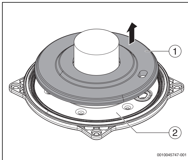
Fig. 64 Desmontar el aislamiento
