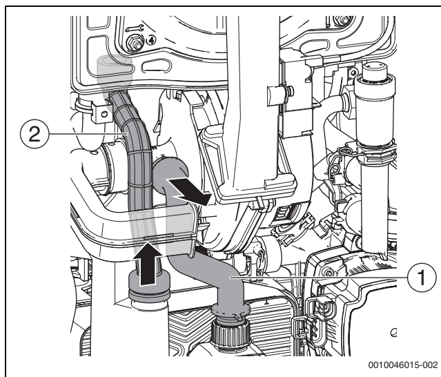
Fig. 109 Desmontar la manguera de evacuación de condensado y la de conexión de gas
