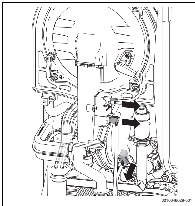
Fig. 112 Desconectar el cable
