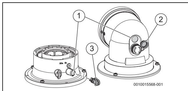
Fig. 33 Punto de medición para la comprobación de la estanqueidad de la tubería de gases de escape
