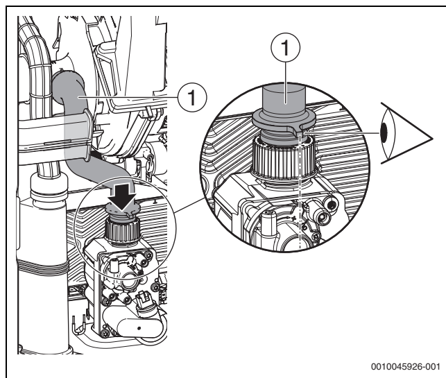
Fig. 122 Colocar y alinear la manguera de conexión de gas
