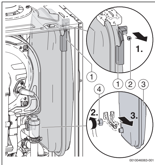
Fig. 134 Desmontar el vaso de expansión
