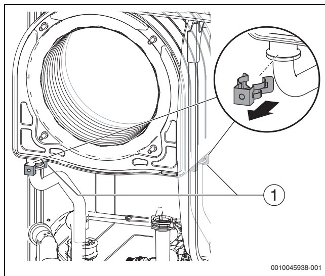
Fig. 99 Desmontar las abrazaderas
