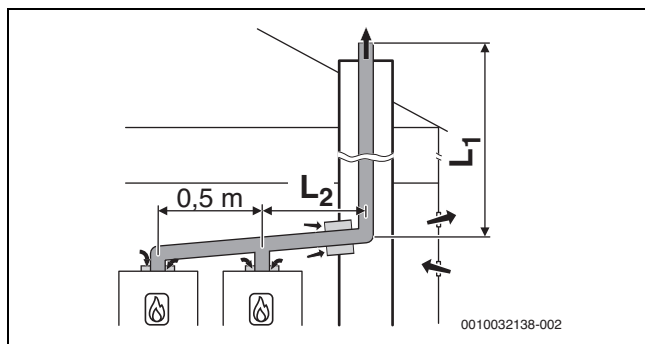
Fig. 19 Sistema en cascada con 2 aparatos: Conducción rígida de gases de evacuación por la chimenea después de B53P con suministro de aire atmosférico en el aparato
