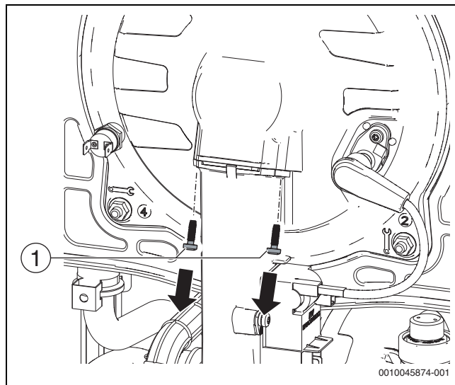
Fig. 123 Desmontaje de los tornillos
