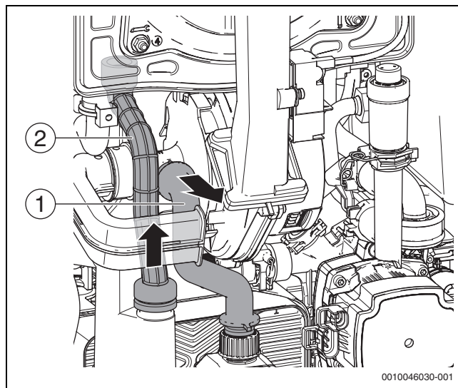
Fig. 113 Retirar la manguera de condensados y de gas
