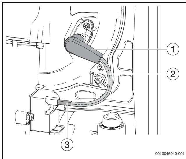
Fig. 127 Sustituir el cable de encendido
