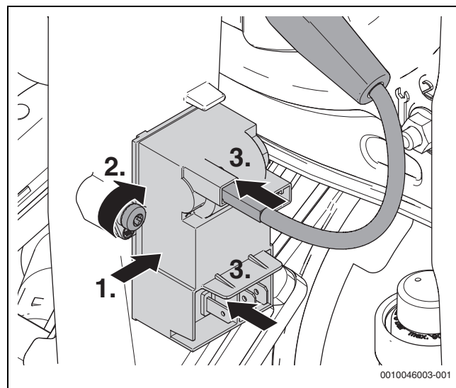
Fig. 106 Instalar el nuevo transformador de encendido
