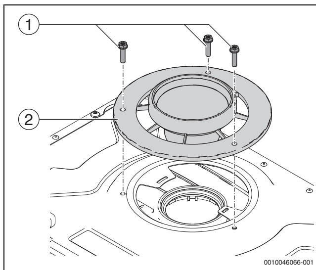
Fig. 57 Desmontar el set y el adaptador del tubo de gases de escape
