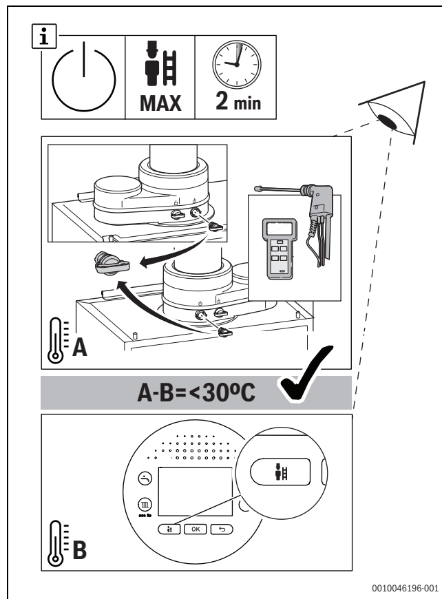
Fig. 74 Prueba de control dT
