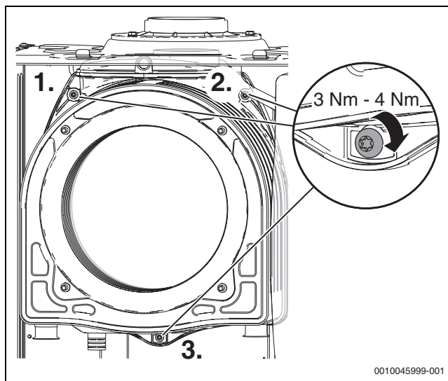
Fig. 103 Instalar el intercambiador de calor nuevo
