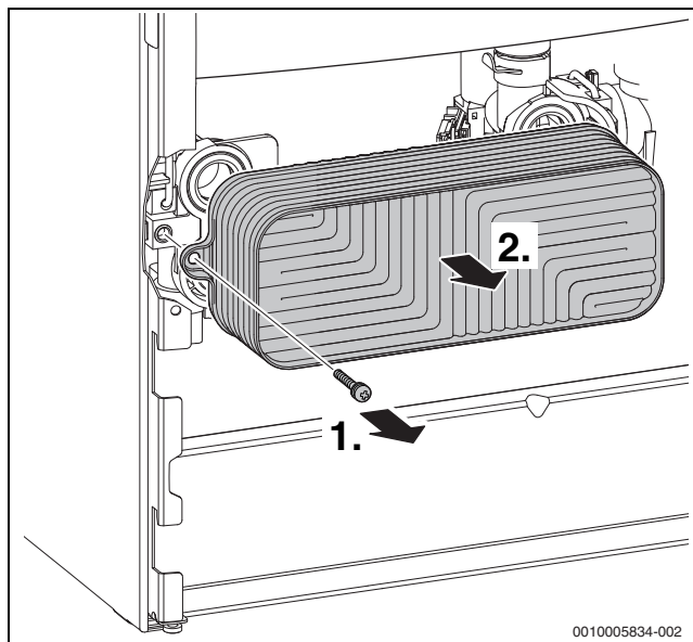
Fig. 140 Desmontar el intercambiador de placas
