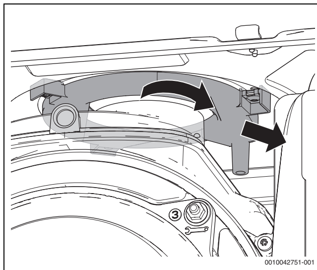
Fig. 148 Desmontar la protección contra la lluvia
