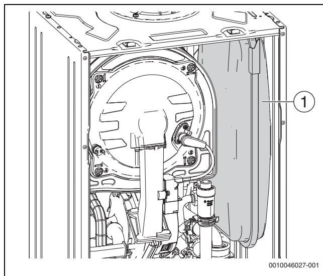
Fig. 62 Comprobar el vaso de expansión
